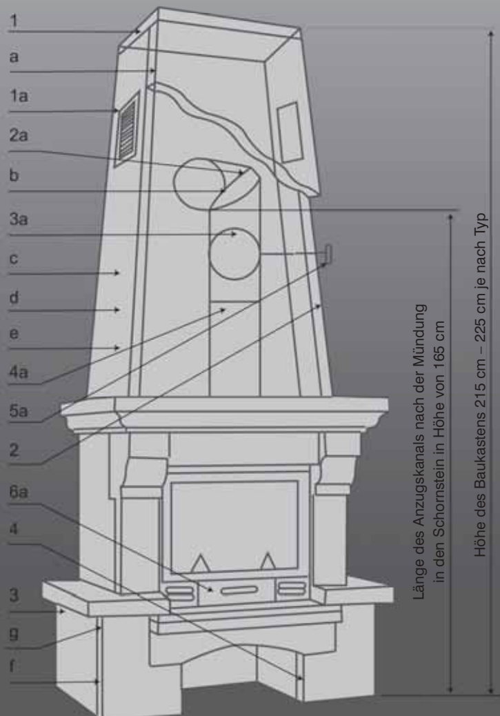
Schema der Baukastenverkleidungen
