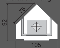
Eckausführung
